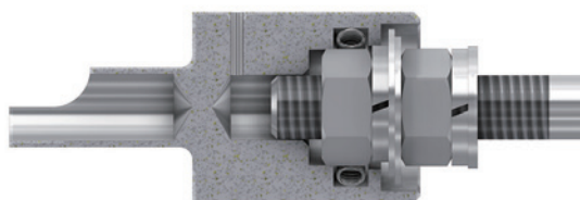
M8ナットの側面接続 5A 24V
